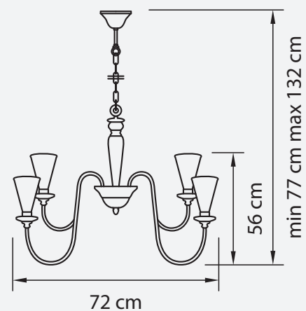
ЛЮСТРА ПОДВЕСНАЯ ● 5,2 kg ⌀ 10 x G9 max 40W
