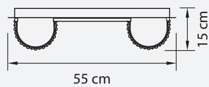
ЛЮСТРА ПОТОЛОЧНАЯ ● 9 kg ⦿ 7 x G9 max 40W
