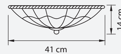
ЛЮСТРА ПОТОЛОЧНАЯ ● 4,5 kg ⦿ 4 x E14 max 60W
