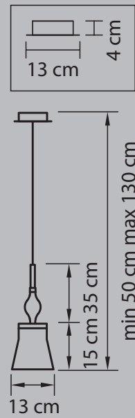
ЛЮСТРА ПОДВЕСНАЯ ● 1,5 kg ⦿ 1 x E14 max 40W
