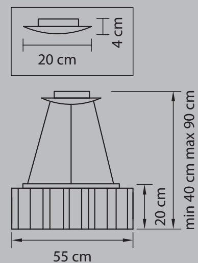
ЛЮСТРА ПОДВЕСНАЯ ● 9,5 kg ⦿ 6 x E27 max 40W
