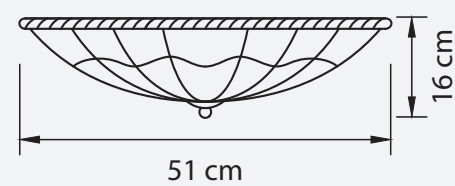
ЛЮСТРА ПОТОЛОЧНАЯ ● 8 kg ⦿ 6 x E14 max 60W
