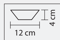
ЛЮСТРА ПОДВЕСНАЯ ● 1,5 kg ⦿ 1 x G9 max 40W
