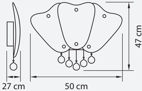
БРА ● 1 kg ⌀ 2 x G9 max 40W
