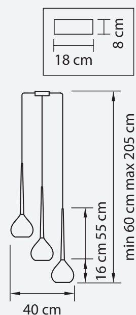
ЛЮСТРА ПОДВЕСНАЯ ● 4,5 kg ⦿ 3 x E14 max 40W
