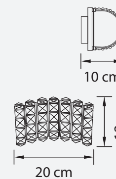
БРА ● 2 kg ⦿ 2 x G9 max 40W
