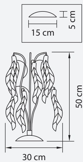
НАСТОЛЬНАЯ ЛАМПА ● 4 kg ○ 3 x G4 12V max 20W
