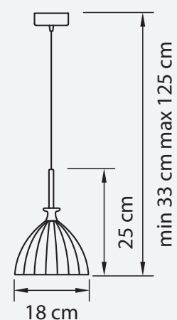
ЛЮСТРА ПОДВЕСНАЯ ● 1 kg ⦿ 1 x E14 max 40W
