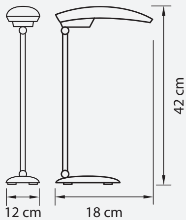
НАСТОЛЬНАЯ ЛАМПА ● 0,9 kg ○ LED max 4W 4200K
