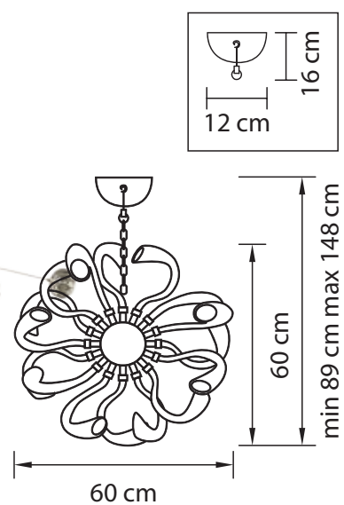
ЛЮСТРА ПОДВЕСНАЯ ● 12 kg ⦿ 12 x G9 max 25W
