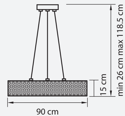
ЛЮСТРА ПОДВЕСНАЯ ● 6,1 kg ⦿ 6 x G9 max 40W
