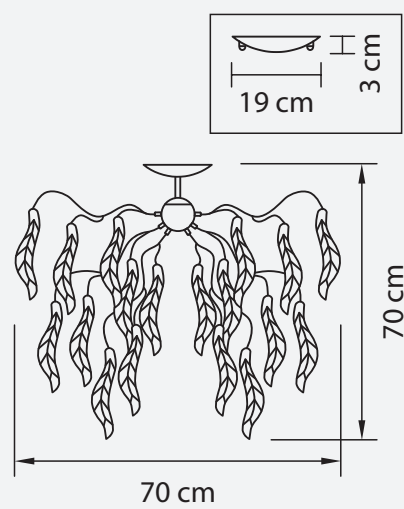
ЛЮСТРА ПОТОЛОЧНАЯ ● 6,5 kg ⦿ 12 x G9 max 40W
