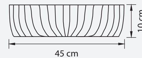
ЛЮСТРА ПОТОЛОЧНАЯ ● 8,5 kg ⦿ 6 x E14 max 60W
