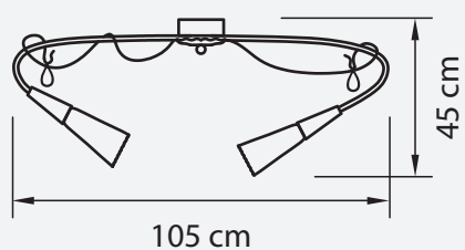
ЛЮСТРА ПОТОЛОЧНАЯ ● 6 kg ○ 12 x G9 max 25W
