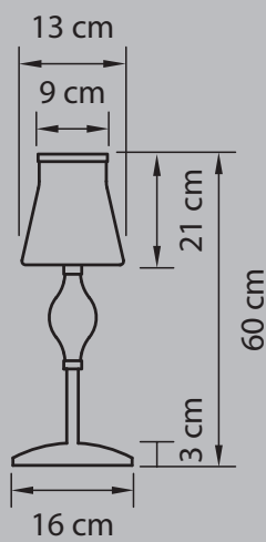
НАСТОЛЬНАЯ ЛАМПА ● 2,5 kg ⦿ 1 x E14 max 40W
