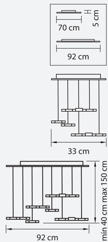
ЛЮСТРА ПОДВЕСНАЯ ● 9 kg ◐ LED 4200K 80W
