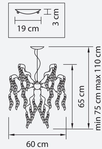
ЛЮСТРА ПОДВЕСНАЯ ● 5 kg ⦿ 9 x G9 max 40W
