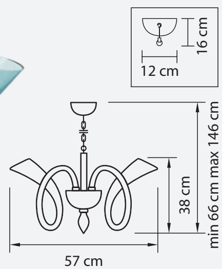
ЛЮСТРА ПОДВЕСНАЯ ● 5,5 kg ⦿ 6 x G9 LED 6W
