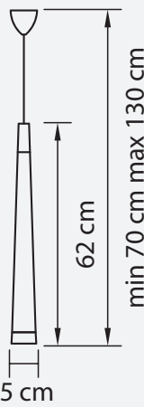
ЛЮСТРА ПОДВЕСНАЯ ● 1,5 kg ⦿ 1 x G9 max 40W
