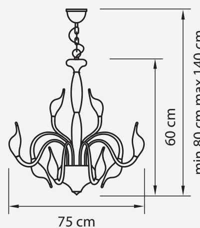
ЛЮСТРА ПОДВЕСНАЯ ● 12 kg ⦿ 12 x G4 12V max 20W
