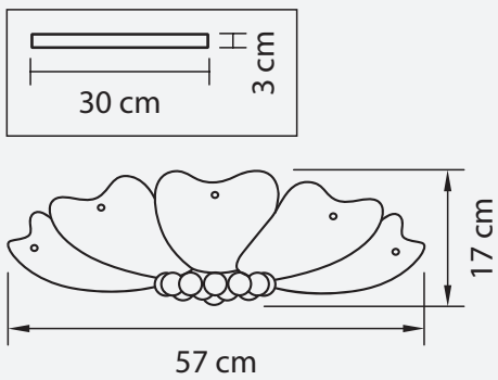
ЛЮСТРА ПОТОЛОЧНАЯ ● 4 kg ⌀ 6 x G9 max 40W
