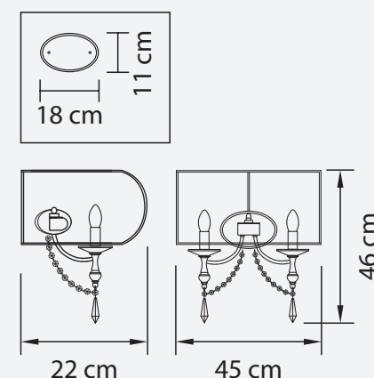
БРА ● 2,5 kg ○ 2 x E14 max 40W
