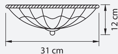
ЛЮСТРА ПОТОЛОЧНАЯ ● 3 kg ⦿ 3 x E14 max 60W
