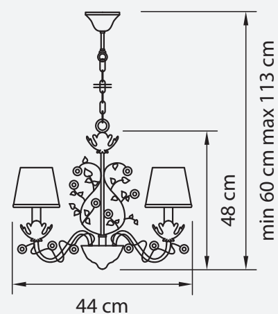
ЛЮСТРА ПОДВЕСНАЯ ● 2,3 kg ⦿ 3 x E14 max 40W
