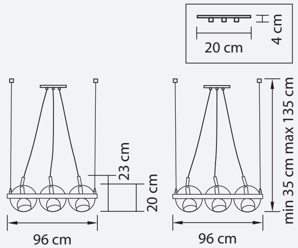
ЛЮСТРА ПОДВЕСНАЯ ● 13 kg ○ 9 x E14 max 40W
