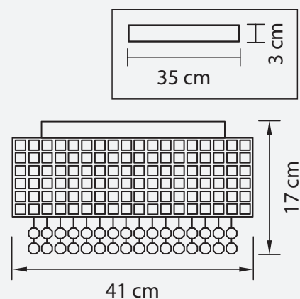
ЛЮСТРА ПОТОЛОЧНАЯ ● 4 kg ⦿ 6 x G9 max 40W
