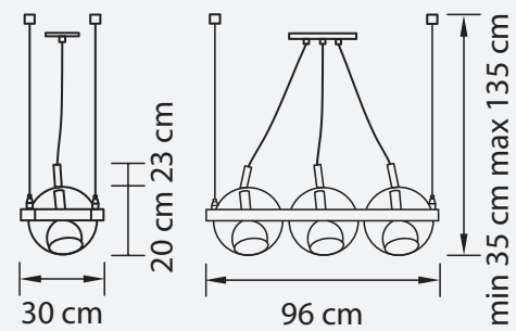
ЛЮСТРА ПОДВЕСНАЯ ● 5 kg ○ 3 x E14 max 40W
