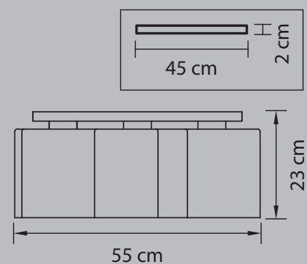
ЛЮСТРА ПОТОЛОЧНАЯ ● 12,5 kg ⦿ 7 x E27 max 40W
