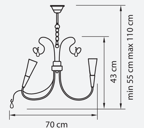
ЛЮСТРА ПОДВЕСНАЯ ● 3,5 kg ⌀ 9 x G9 max 25W
