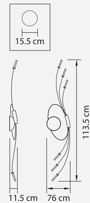
БРА ● 1,6 kg ⦿ 6 x G4 12v max 20W
