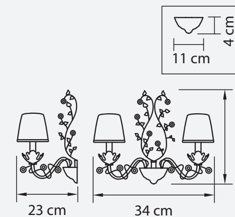
БРА ● 1,1 kg ⦿ 2 x E14 max 40W
