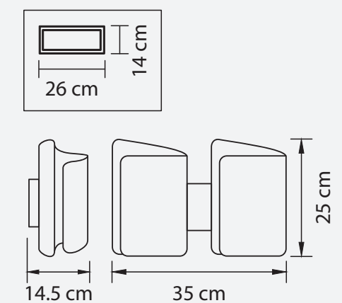
БРА ● 3 kg ⦿ 2 x E27 max 40W
