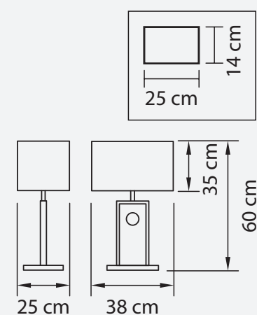
НАСТОЛЬНАЯ ЛАМПА ● 4 kg ⦿ 1 X E27 MAX 60W
