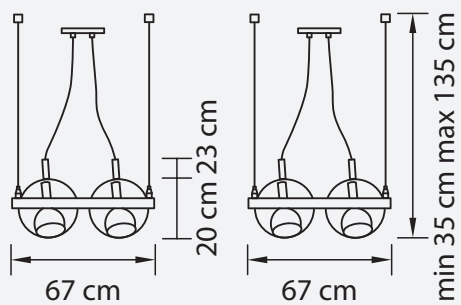
ЛЮСТРА ПОДВЕСНАЯ ● 6 kg ○ 4 x E14 max 40W
