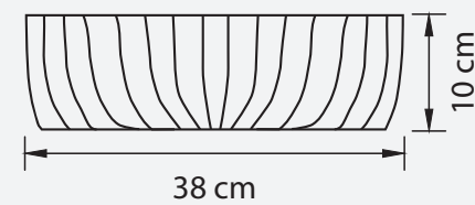
ЛЮСТРА ПОТОЛОЧНАЯ ● 9,5 kg ⦿ 4 x E14 max 60W
