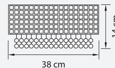
БРА ● 1,5 kg ⦿ 2 x G9 max 40W
