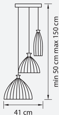
ЛЮСТРА ПОДВЕСНАЯ ● 5 kg ⦿ 3 x E14 max 40W
