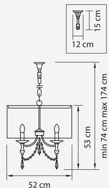
ЛЮСТРА ПОДВЕСНАЯ ● 4,5 kg ○ 3 x E14 max 40W
