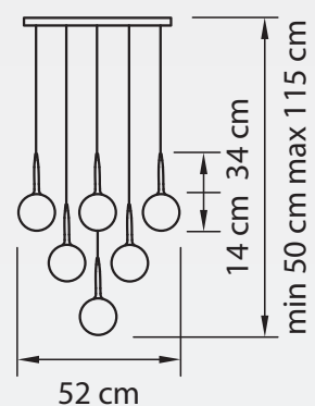
ЛЮСТРА ПОДВЕСНАЯ ● 10 kg ⦿ 10 x G9 max 40W
