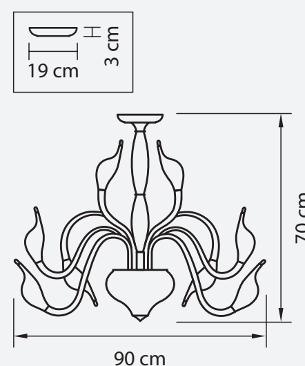
ЛЮСТРА ПОТОЛОЧНАЯ ● 16 kg ⦿ 18 x G4 12V max 20W
