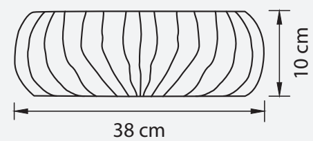
ЛЮСТРА ПОТОЛОЧНАЯ ● 6,5 kg ⦿ 4 x E14 max 60W
