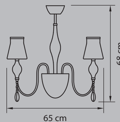
ЛЮСТРА ПОТОЛОЧНАЯ ● 8,5 kg ○ 5 x E14 max 40W ○ 1 x G9 max 40W
