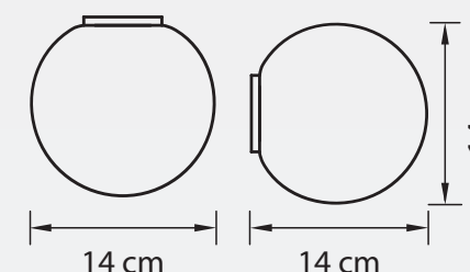
БРА/ПОТОЛОЧНЫЙ СВЕТИЛЬНИК ● 1 kg ⦿ 1 x G9 max 40W
