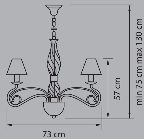
ЛЮСТРА ПОДВЕСНАЯ ● 7 kg ⦿ 9 x E14 max 40W
