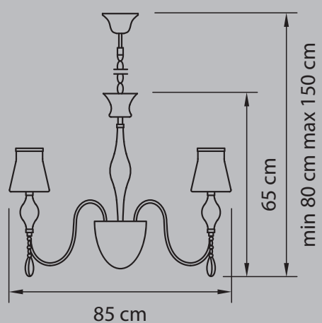
ЛЮСТРА ПОДВЕСНАЯ ● 11 kg ○ 8 x E14 max 40W ○ 1 x G9 max 40W
