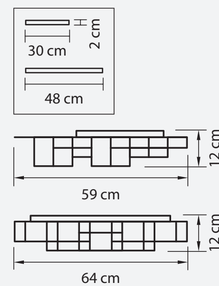
ЛЮСТРА ПОТОЛОЧНАЯ ● 9 kg ◐ LED 4200K 80W
