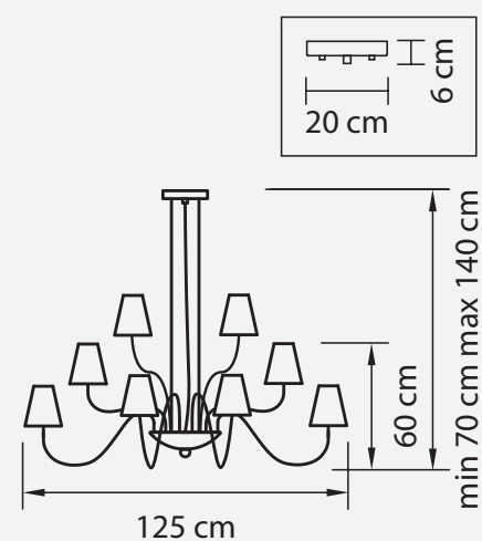
ЛЮСТРА ПОДВЕСНАЯ ● 15 kg ⦿ 21 x G9 max 40W
