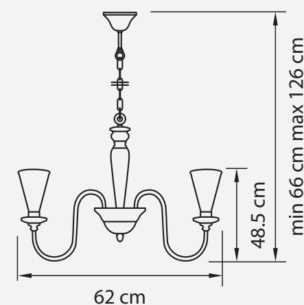
ЛЮСТРА ПОДВЕСНАЯ ● 3,5 kg ⌀ 6 x G9 max 40W
