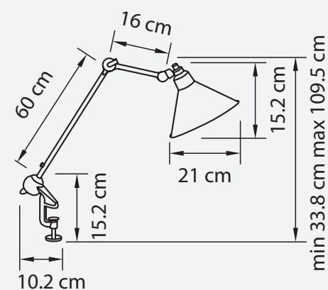
НАСТОЛЬНАЯ ЛАМПА ● 2 kg ⦿ 1 x E14 max 40W
