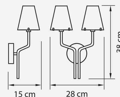
БРА ● 1,2 kg ⌀ 2 x G9 max 40W
