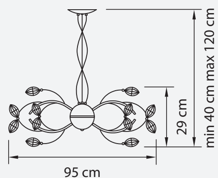
ЛЮСТРА ПОДВЕСНАЯ ● 8 kg ○ 16 x G4 max 20W
