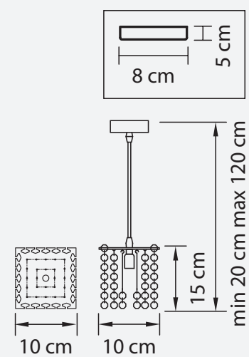
ЛЮСТРА ПОДВЕСНАЯ ● 0,5 kg ⦿ 1 x G9 max 40W
