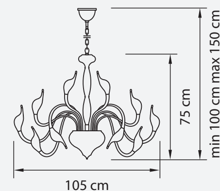
ЛЮСТРА ПОДВЕСНАЯ ● 26 kg ⦿ 24 x G4 12V max 20W
