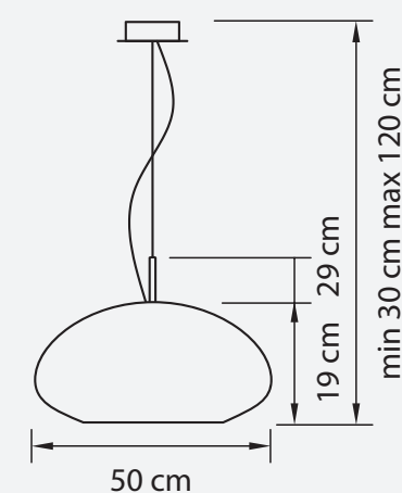
ЛЮСТРА ПОДВЕСНАЯ ● 3 kg ○ 3 x E27 max 40W
