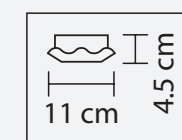
ЛЮСТРА ПОДВЕСНАЯ ● 0,5 kg ⦿ 1 x G9 max 25W
