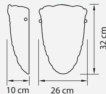
БРА ● 2 kg ⦿ 2 x E14 max 40W
