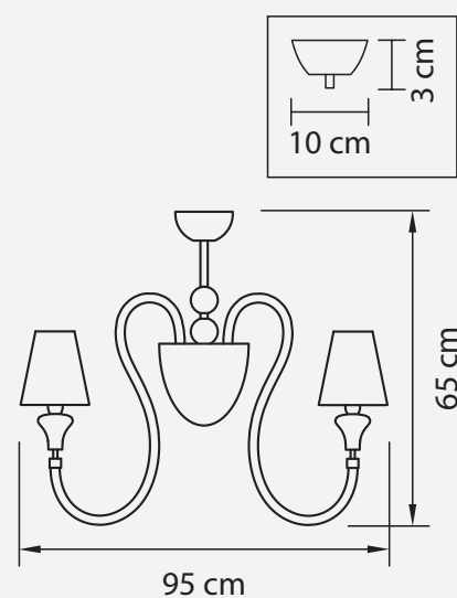
ЛЮСТРА ПОТОЛОЧНАЯ ● 10 kg ⦿ 8 x E14 max 40W ⦿ 1 x G9 max 40W
