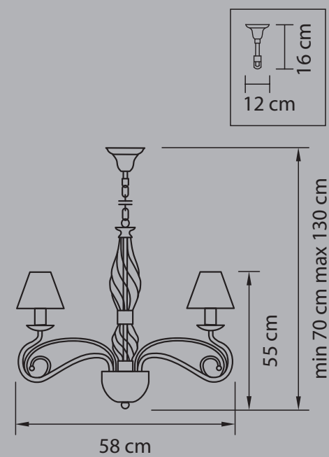
ЛЮСТРА ПОДВЕСНАЯ ● 4 kg ⦿ 6 x E14 max 40W
