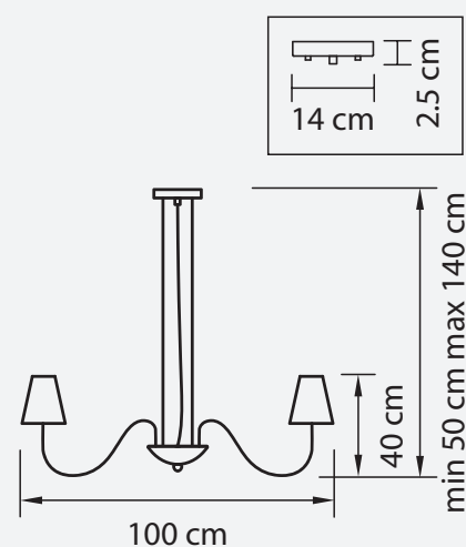
ЛЮСТРА ПОДВЕСНАЯ ● 4 kg ⌀ 8 x G9 max 40W
