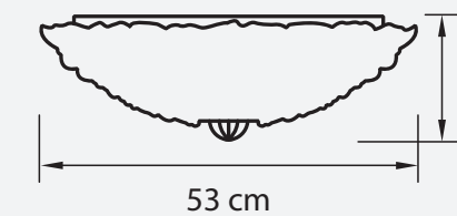
ЛЮСТРА ПОТОЛОЧНАЯ ● 5 kg ⦿ 6 x E14 max 40W
