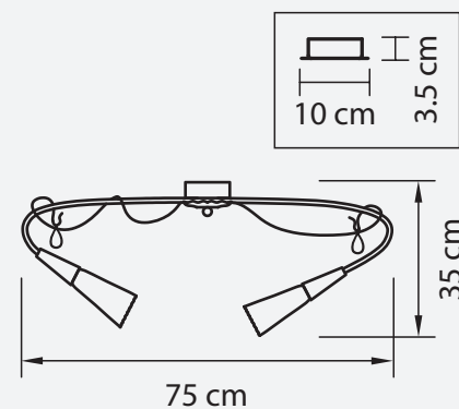
ЛЮСТРА ПОТОЛОЧНАЯ ● 2,5 kg ⌀ 6 x G9 max 25W
