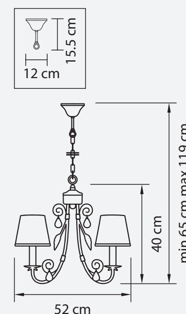
ЛЮСТРА ПОДВЕСНАЯ ● 2,9 kg ⌀ 5 x E14 max 40W
