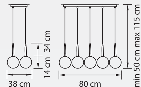
ЛЮСТРА ПОДВЕСНАЯ ● 7,5 kg ⦿ 8 x G9 max 40W
