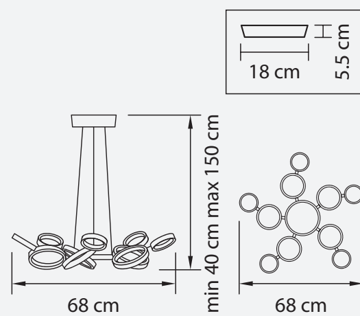
ЛЮСТРА ПОДВЕСНАЯ ● 3 kg ○ LED, max 11,5W, 4000K
