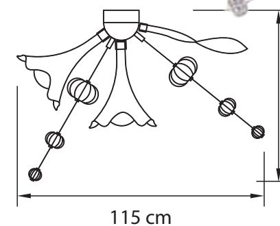
ЛЮСТРА ПОТОЛОЧНАЯ ● 8 kg ⦿ 12 x G9 max 25W
