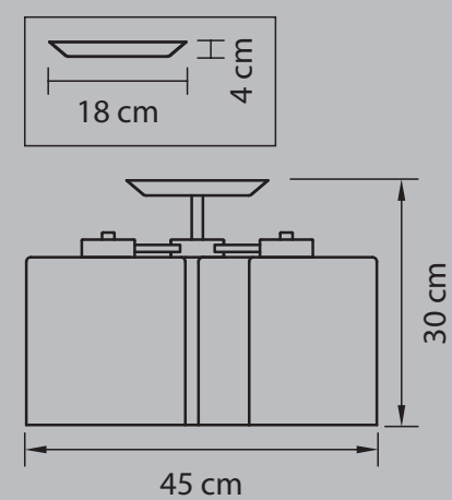
ЛЮСТРА ПОТОЛОЧНАЯ ● 5 kg ⦿ 3 x E27 max 40W
