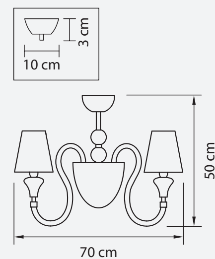
ЛЮСТРА ПОТОЛОЧНАЯ ● 7 kg ⦿ 5 x E14 max ⦿ 1 x G9 max 40W
