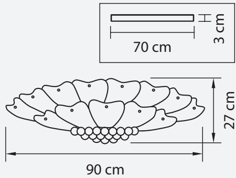
ЛЮСТРА ПОТОЛОЧНАЯ ● 15,5 kg ⌀ 18 x G9 max 40W
