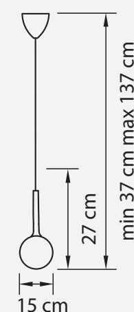
ЛЮСТРА ПОДВЕСНАЯ ● 1 kg ⦿ 1 x E14 max 40W
