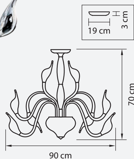
ЛЮСТРА ПОТОЛОЧНАЯ ● 16 kg ⦿ 18 x G4 12V max 20W
