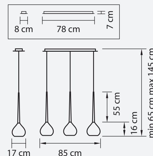
ЛЮСТРА ПОДВЕСНАЯ ● 4,5 kg ⦿ 3 x E14 max 40W
