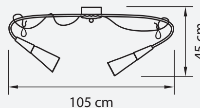
ЛЮСТРА ПОТОЛОЧНАЯ ● 6 kg ○ 12 x G9 max 25W
