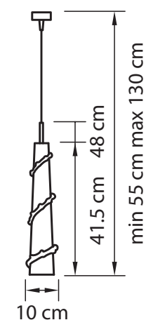
ЛЮСТРА ПОДВЕСНАЯ ● 1,5 kg ○ 1 x E14 max 40W
