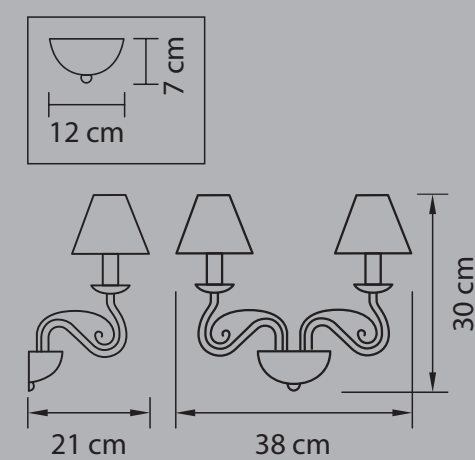
БРА ● 1 kg ⦿ 2 x E14 max 40W
