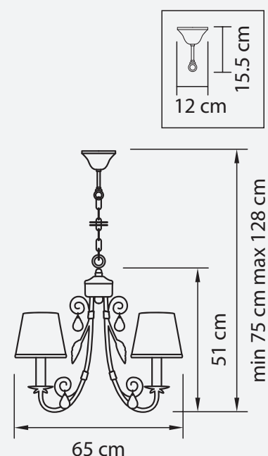
ЛЮСТРА ПОДВЕСНАЯ ● 4,25 kg ⌀ 8 x E14 max 40W
