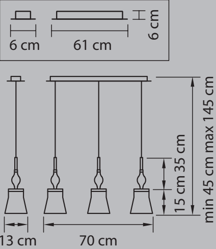
ЛЮСТРА ПОДВЕСНАЯ ● 3,5 kg ⦿ 3 x E14 max 40W
