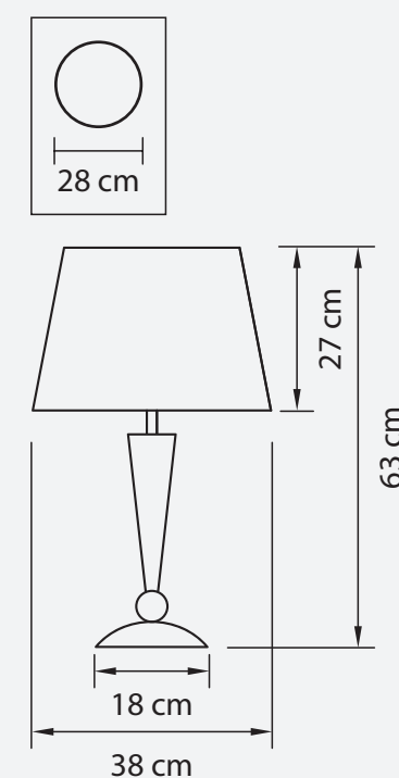
НАСТОЛЬНАЯ ЛАМПА ● 2 kg ⦿ 1 x E27 max 60W
