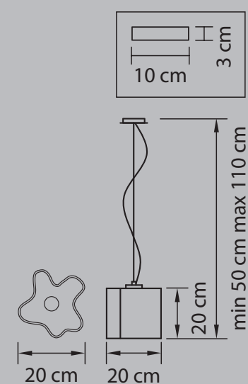
ЛЮСТРА ПОДВЕСНАЯ ● 1,5 kg ⦿ 1 x E27 max 40W
