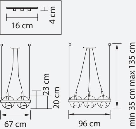
ЛЮСТРА ПОДВЕСНАЯ ● 7,5 kg ○ 6 x E14 max 40W
