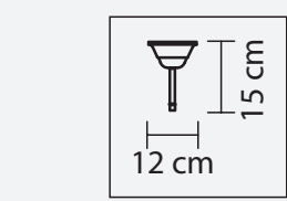
ЛЮСТРА ПОДВЕСНАЯ ● 3,5 kg ⌀ 9 x G9 max 25W
