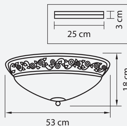
ЛЮСТРА ПОТОЛОЧНАЯ ● 3,8 kg ⦿ 3 x E27 max 40W
