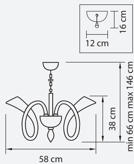
ЛЮСТРА ПОДВЕСНАЯ ● 6,5 kg ⦿ 8 x G9 LED 6W
