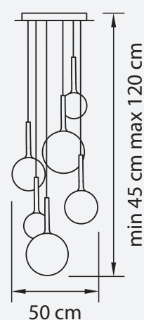
ЛЮСТРА ПОДВЕСНАЯ ● 11 kg ⦿ 6 x E14 max 40W
