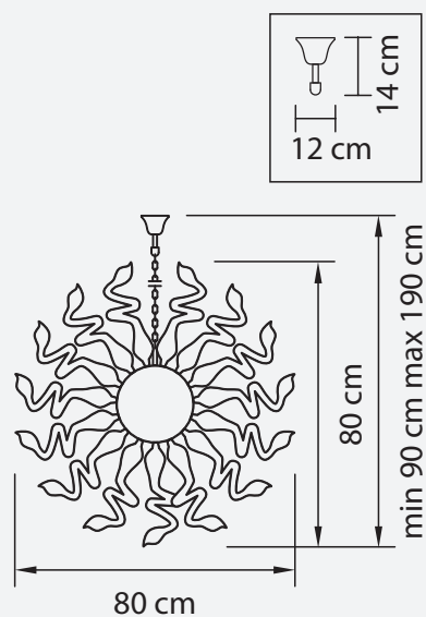
ЛЮСТРА ПОДВЕСНАЯ ● 25 kg ⦿ 18 x G9 max 40W
