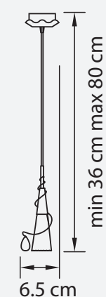
ЛЮСТРА ПОДВЕСНАЯ ● 0,5 kg ⦿ 1 x G9 max 25W
