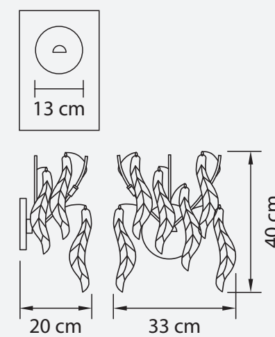
БРА ● 1 kg ⦿ 3 x G4 12V max 20W
