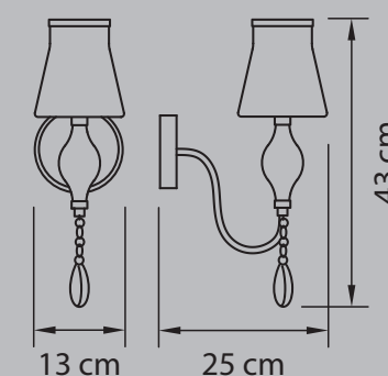
БРА ● 1,5 kg ○ 1 x E14 max 40W
