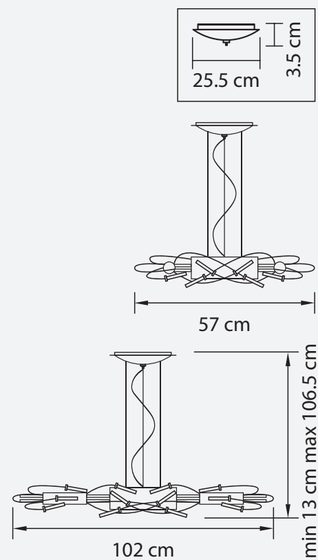
ЛЮСТРА ПОДВЕСНАЯ ● 8,3 kg ⦿ 24 x G4 12v max 20W
