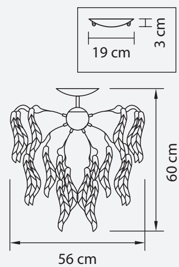
ЛЮСТРА ПОТОЛОЧНАЯ ● 4,5 kg ⦿ 9 x G9 max 40W
