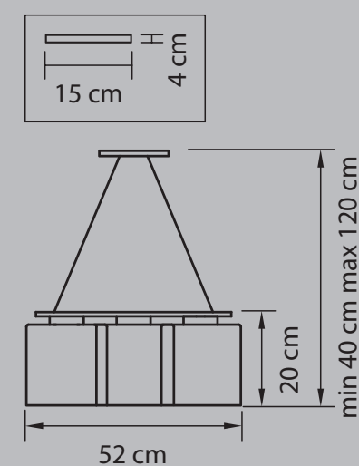
ЛЮСТРА ПОДВЕСНАЯ ● 4 kg ⦿ 3 x E27 max 40W
