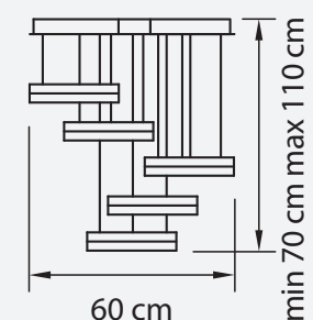
ЛЮСТРА ПОДВЕСНАЯ ● 11 kg ○ LED, max 46W, 4000K
