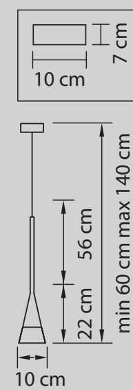
ЛЮСТРА ПОДВЕСНАЯ ● 1 kg ⦿ 1 x E14 max 40W
