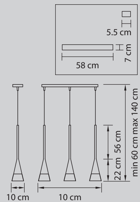
ЛЮСТРА ПОДВЕСНАЯ ● 4 kg ⦿ 3 x E14 max 40W
