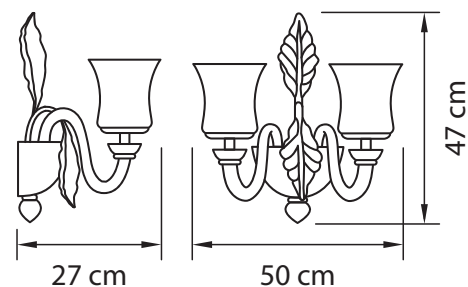
БРА ● 3,5 kg ○ 2 x E14 max 40W
