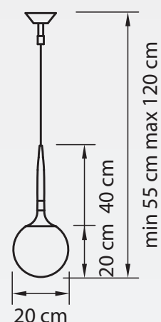
ЛЮСТРА ПОДВЕСНАЯ ● 1,5 kg ⦿ 1 x G9 max 40W
