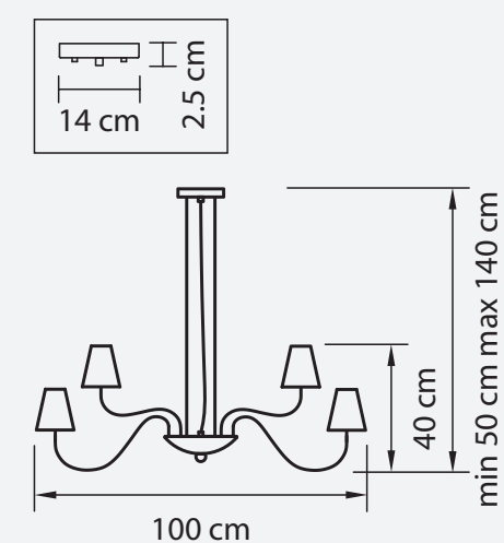
ЛЮСТРА ПОДВЕСНАЯ ● 9 kg ⦿ 16 x G9 max 40W
