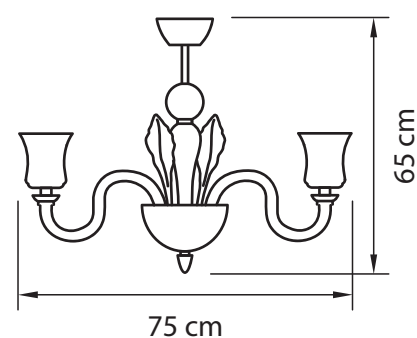
ЛЮСТРА ПОТОЛОЧНАЯ ● 12 kg ○ 6 x E14 max 40W
