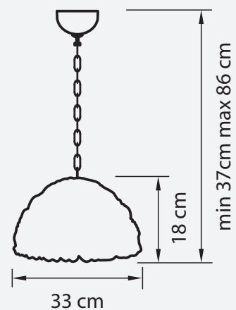
ЛЮСТРА ПОДВЕСНАЯ ● 4 kg ⦿ 1 x E27 max 40W
