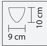
ЛЮСТРА ПОДВЕСНАЯ ● 1,5 kg ⦿ 1 x G9 max 40W
