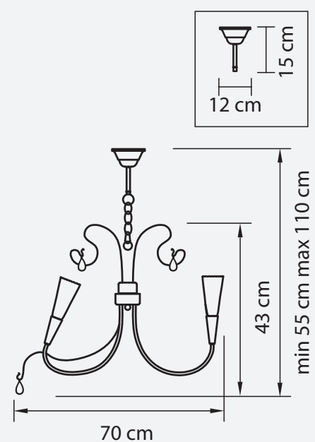
ЛЮСТРА ПОДВЕСНАЯ ● 3,5 kg ⦿ 9 x G9 max 25W
