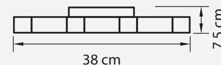
ЛЮСТРА ПОТОЛОЧНАЯ ● 2,5 kg ◐ LED 4200K 35W
