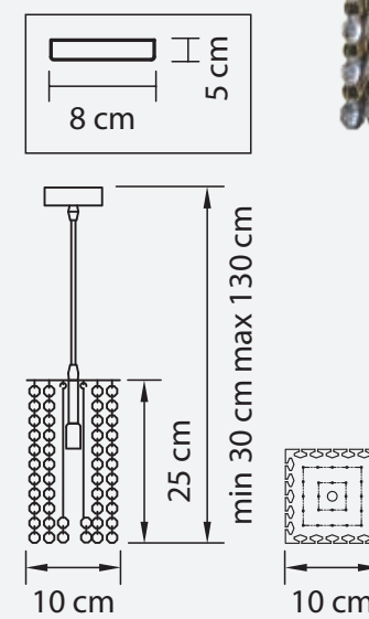
ЛЮСТРА ПОДВЕСНАЯ ● 0,8 kg ⦿ 1 x G9 max 40W
